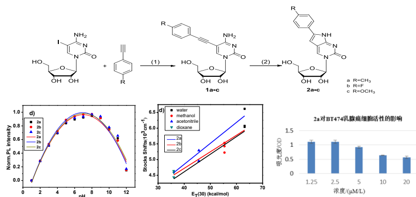
图 2 核苷类化合物的合成及其荧光探针性能与抗肿瘤活性示例图
