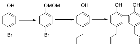
图 4 厚朴与厚朴酚的制备路线图
