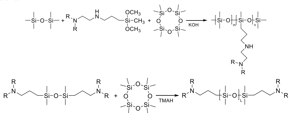
图 3 柔顺剂与氨基硅油的制备路线图
