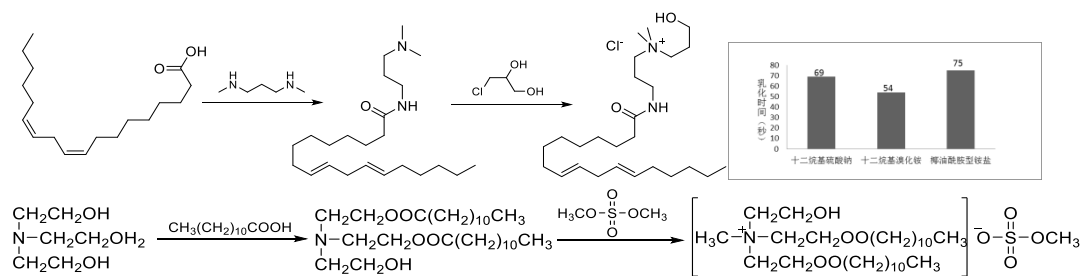
图 5 天然油脂表面活性剂的制备与性能示例图
