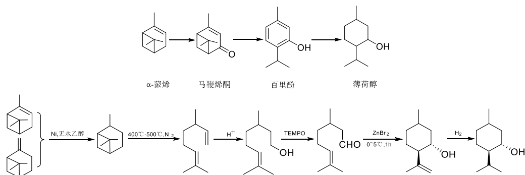
图 1 薄荷与薄荷醇的制备路线示例图
